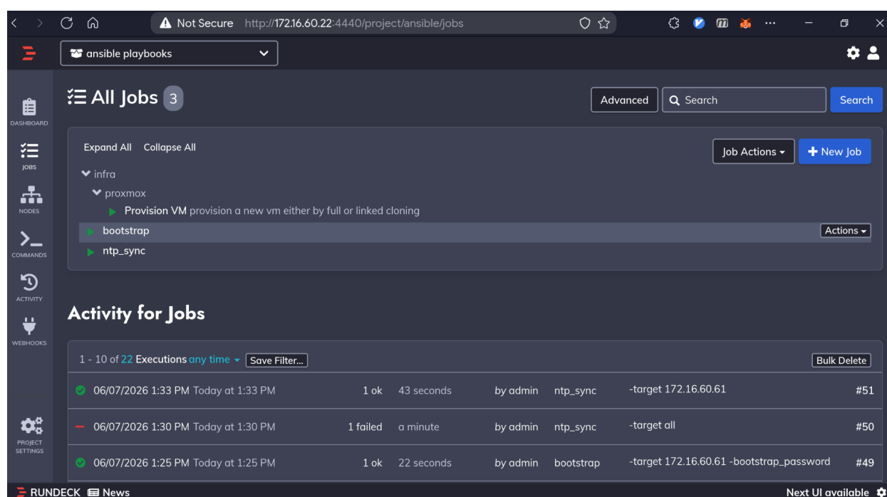
FIGURE IV.68 – Interface Rundeck affichant les jobs de provisionnement Ansible.
