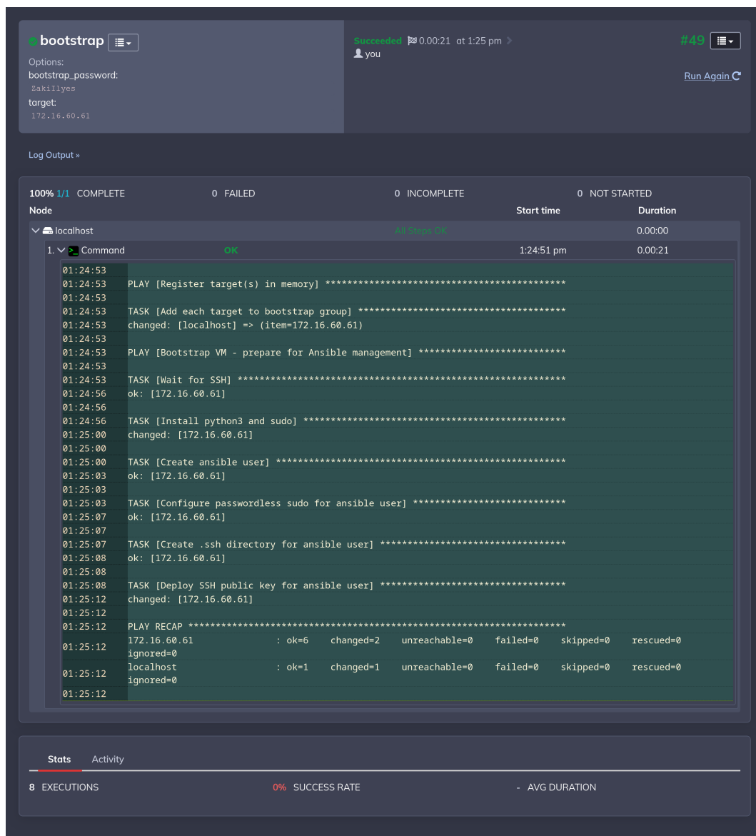
FIGURE C.1 – Résultat d'exécution d'un job Rundeck avec le journal Ansible complet.
