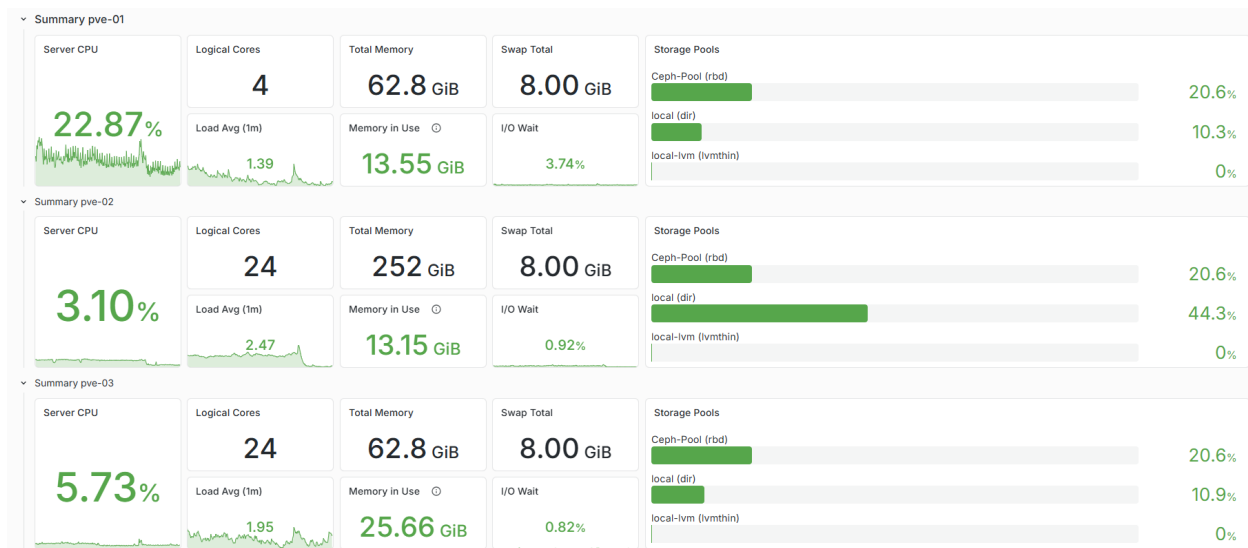
FIGURE IV.17 – Dashboard Grafana Infrastructure pour les nœuds Proxmox.
