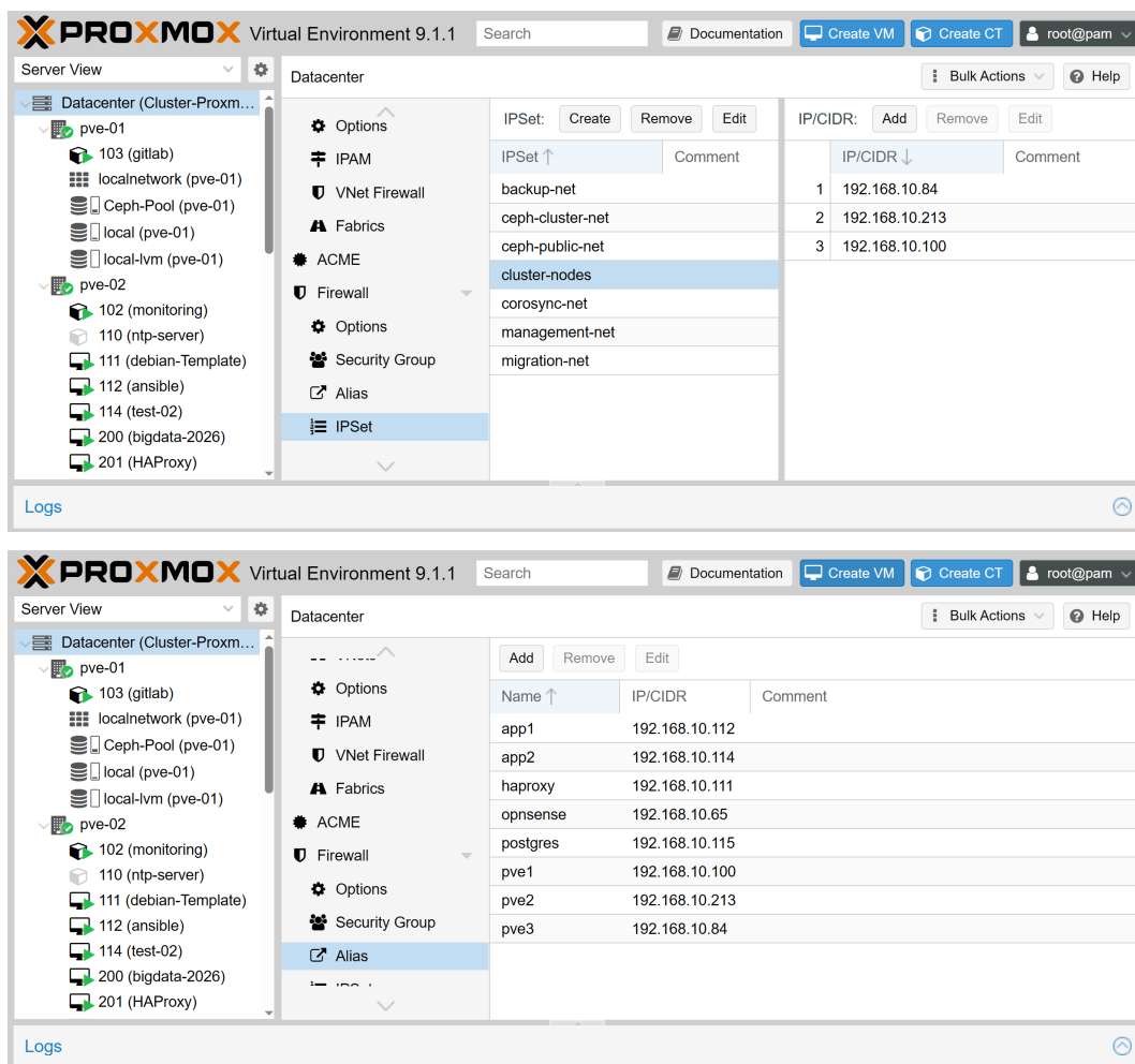
FIGURE D.2 – IPSets et alias configurés au niveau datacenter dans le pare-feu Proxmox.
