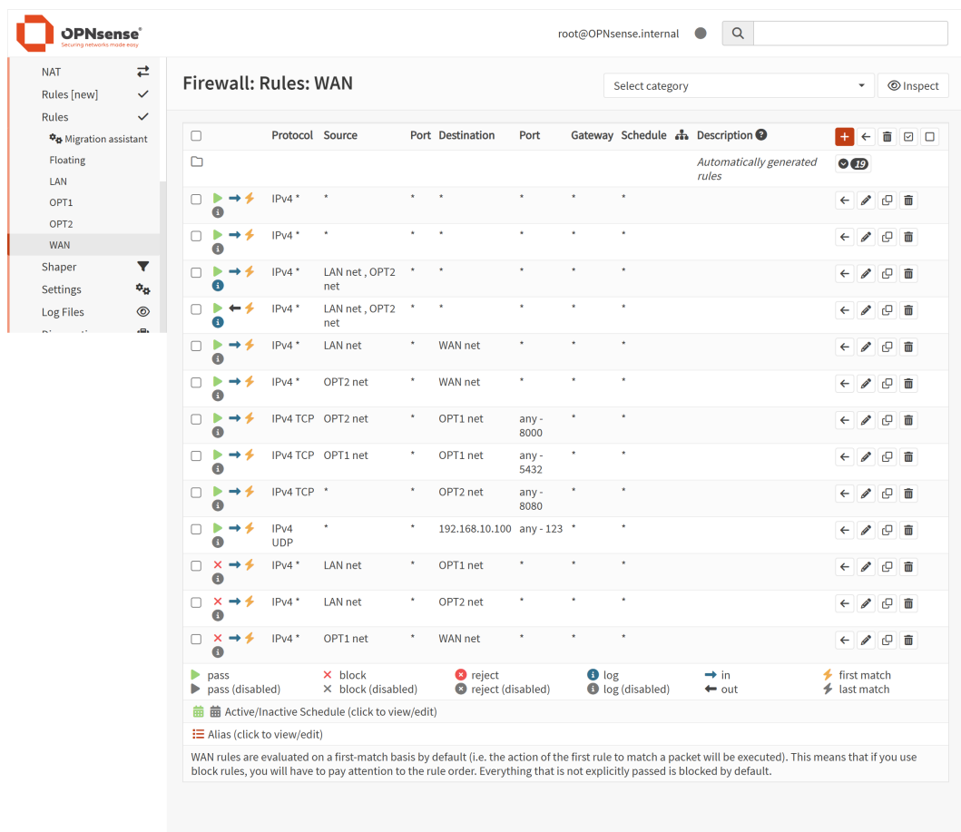
FIGURE D.1 – Règles de filtrage inter-zones dans l'interface OPNsense (Firewall -> Rules).
